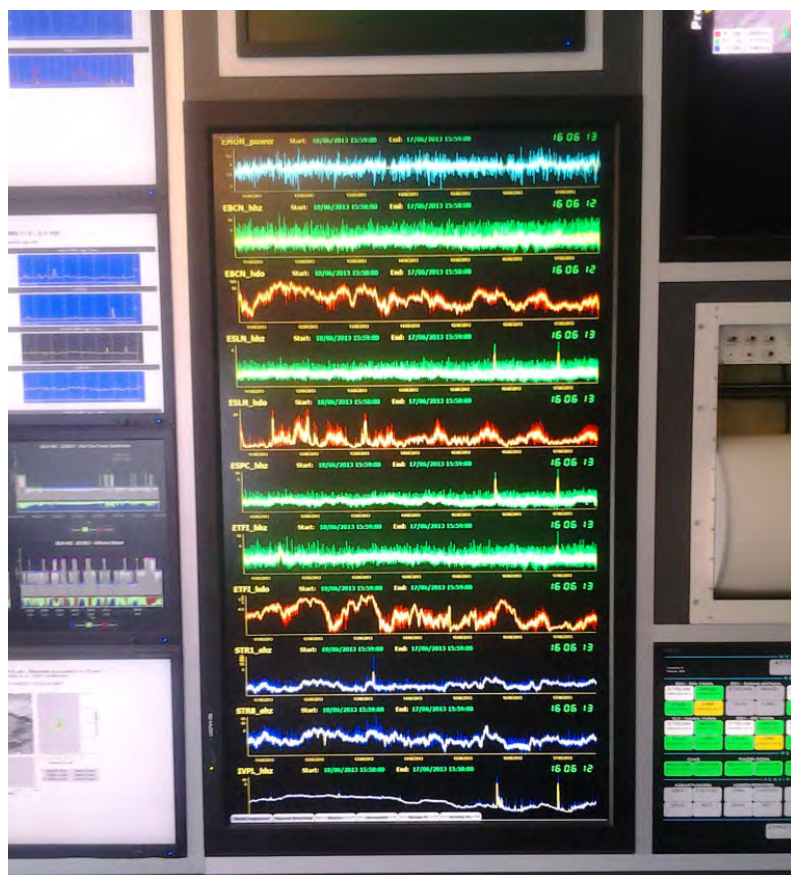
Figura 20. Applicativo TSViewer in funzione nella Sala Operativa dell'Osservatorio Etneo. I differenti colori delle serie sono relative alla tipologia di dato visualizzata; in azzurro il segnale del radar ubicato al sito La Montagnola; in verde l'ampiezza del tremore vulcanico; in rosso l'RMS del segnale infrasonico; in blu l'RMS del segnale sismico relativo a tre stazioni delle Eolie.
