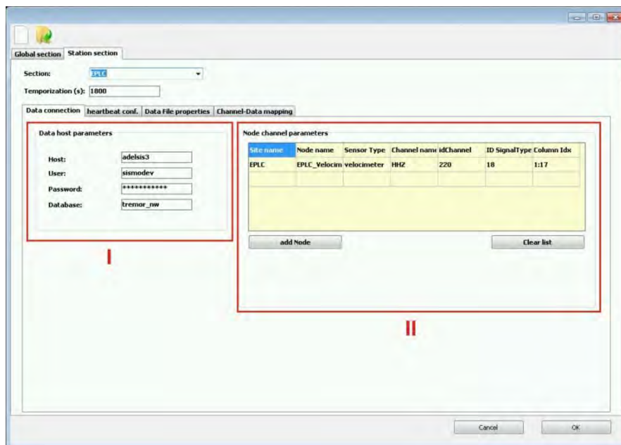
Figura 13. Dettaglio della sotto-sezione Data connection .
