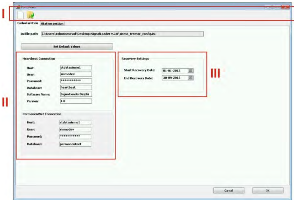
Figura 12. Sezione Global section del programma di configurazione.
