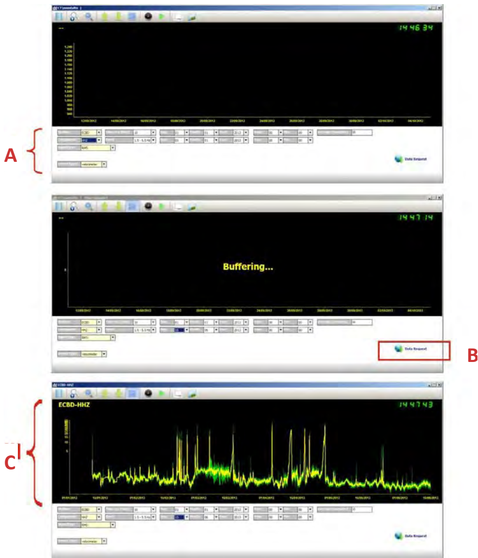
Figura 19. Richiesta del dato: A) Impostazione dei parametri nel pannello III; B) invio della richiesta a TSDSsystem ; C) la serie temporale è visibile nel pannello II.
