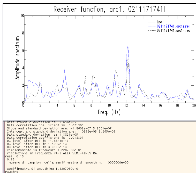
Figura 7. L'output su schermo della macro receiver consiste nel rapporto spettrale EW/V e NS/V.
