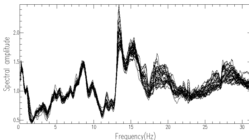
Figura 11. Rapporti spettrali medi orari H/V durante un'intera giornata.
