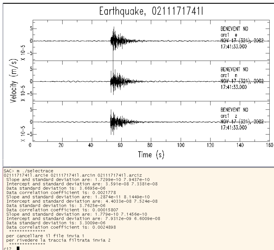
Figura 4. Schermata della macro selecttrace.
