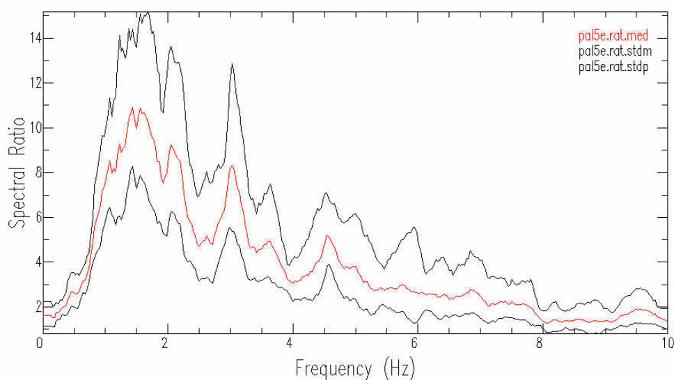
Figura 10. Media +/- deviazione standard di 18 rapporti spettrali della componente EW rispetto a un sito di riferimento. La stazione si trova nella città di Palermo.
