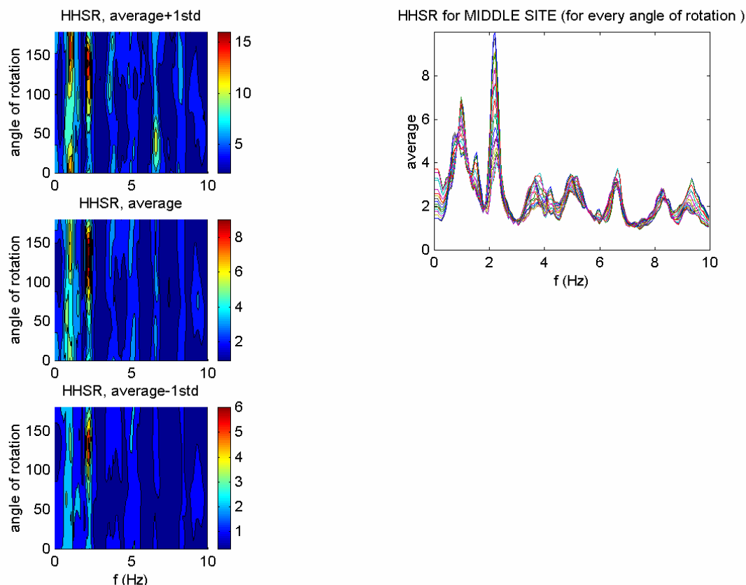
Figura 9. Destra) La media dei classici rapporti spettrali H/Hrif ottenuta nel bacino di Colfiorito. Ogni curva corrisponde ad una rotazione di 10° in senso orario del nord. Sinistra) I valori della media, della media + la deviazione standard, e della media – la deviazione standard sono stati plottati in funzione della frequenza e dell'angolo di rotazione. In questo caso si evidenzia bene una forte direzionalità dell'amplificazione a 2.25 HZ, con il massimo in direzione N130°.
