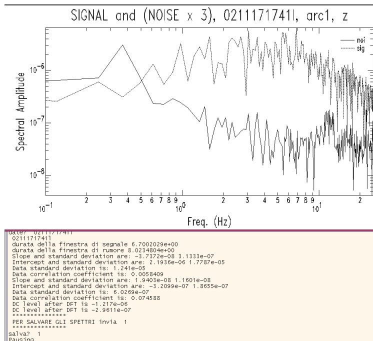
Figura 6. Confronto fra lo spettro di segnale e quello di rumore moltiplicato per tre.
