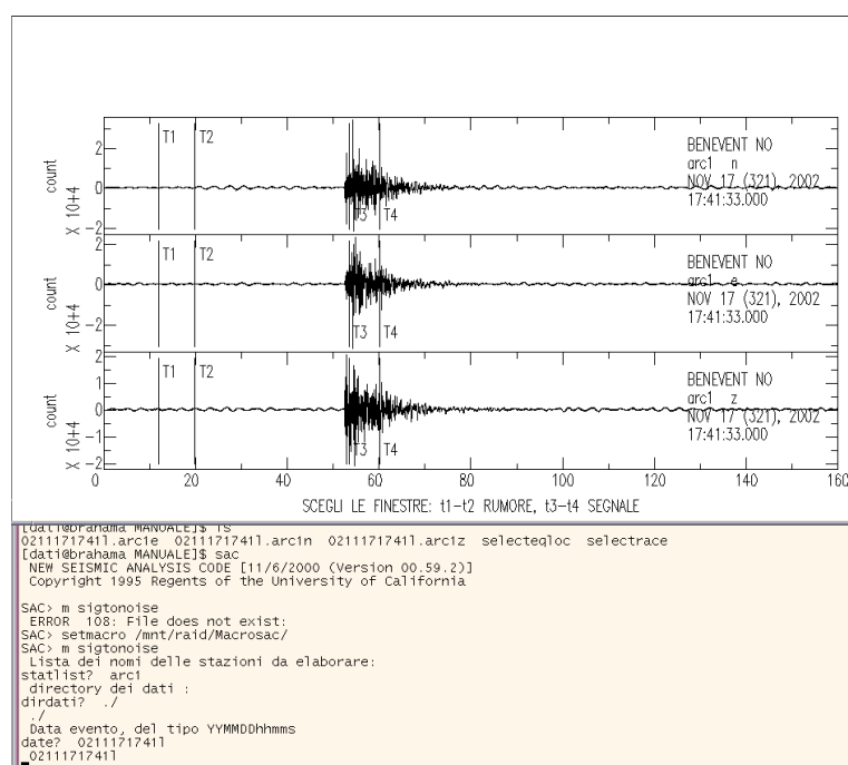
Figura 5. Scelta delle finestre di segnale e rumore tramite la macro sigtonoise.
