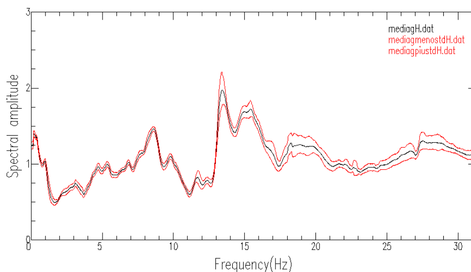
Figura 12. Media giornaliera \pm deviazioni standard per i files H/V orari di figura 11.
