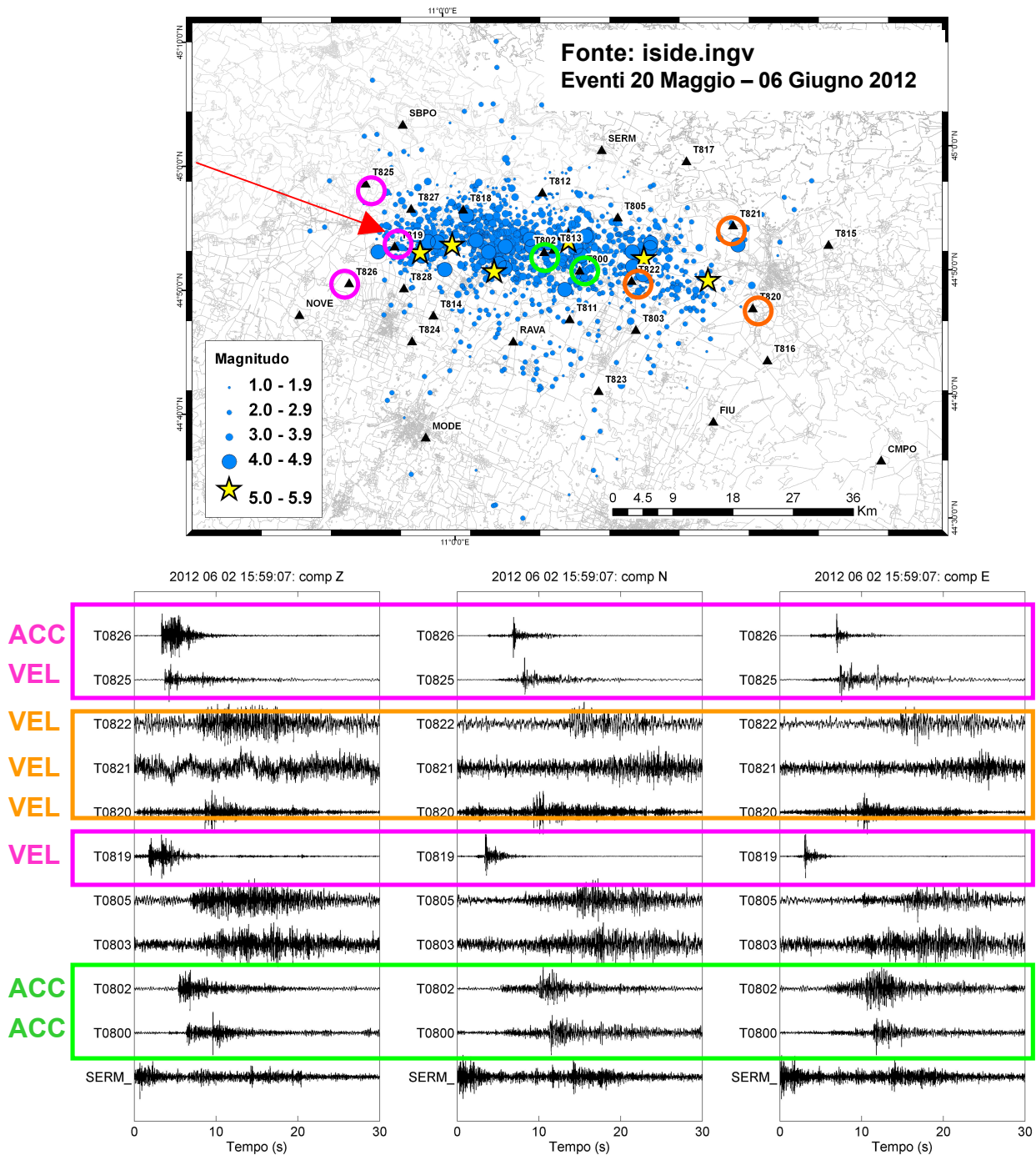
Figura 13. Evento di M_L 2.5 e profondità 25.3 Km [Fonte Dati: ISIDe; Mele et al. 2007; 2011] in area occidentale rispetto alla sequenza, registrato dalle stazioni della rete di pronto intervento INGV trasmesse in real-time . La freccia rossa indica la posizione dell'epicentro dell'evento.
